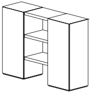
150 x 43 Höhe height 110
